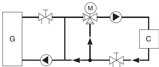
Рис. 12: Радиаторный контур подключенный к котельной тепловой установки
