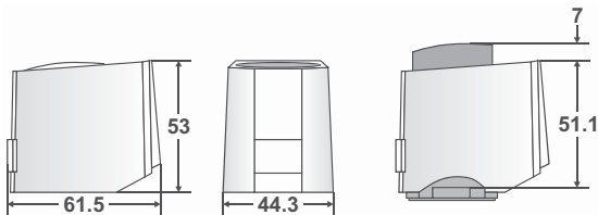
Габаритные размеры в мм
