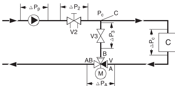
Рис. 3: 3-х ходовой смесительный клапан
