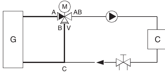
Рис. 7: Трех-ходовой смешивательный клапан
