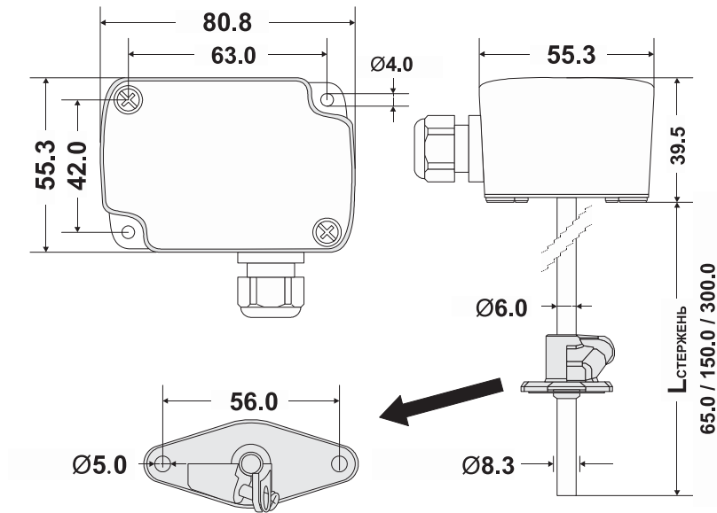
Рис. 1. Габаритные размеры датчика температуры в мм
