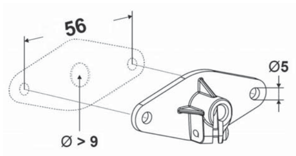
Рис. 2. Габаритные размеры монтажного фланца в мм
