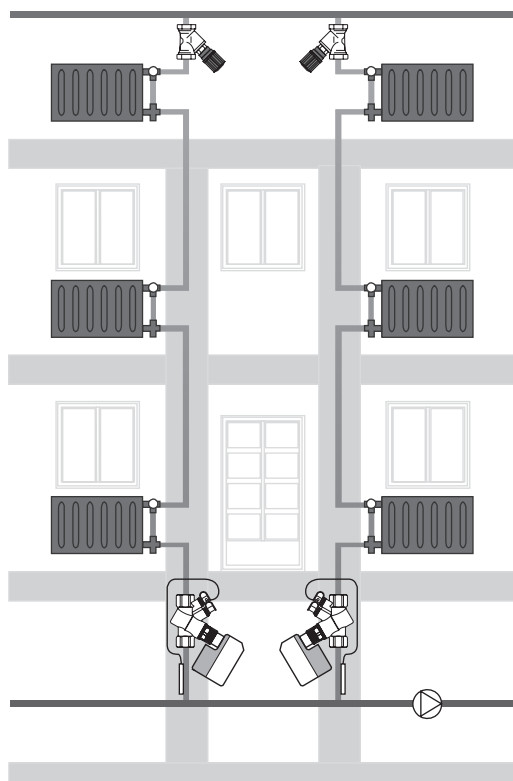
Рис. 5 Отопление, 1-трубная вертикальная система
