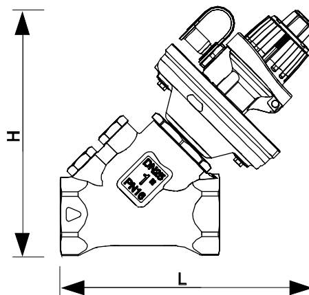
Рис. 2 Вид сбоку
