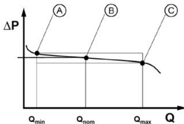
Рис. 6 Регулирующая характеристика
